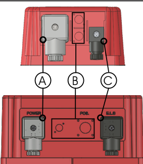
A Versorgungsstecker B Optional C Endlagenstecker
